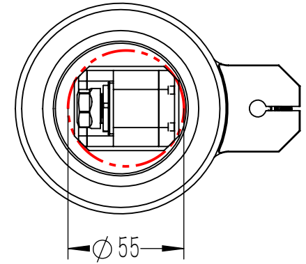
铣头参数表
